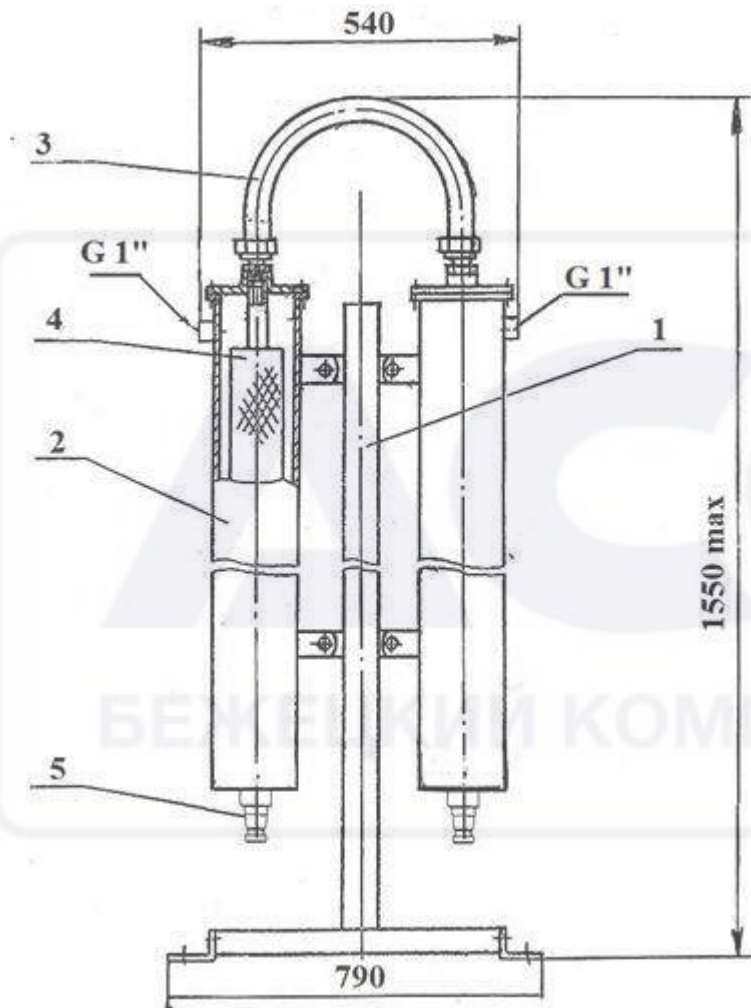
Рис. 2 Фильтрационный модуль ФМ-180/16Ц; ФМ-300/16Ц
